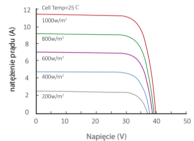
Krzywa prądowo-napięciowa (LR4-60HIH-365M)
