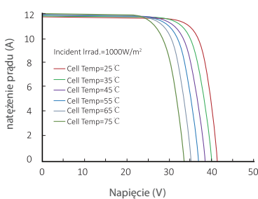
Krzywa prądowo-napięciowa (LR4-60HIH-365M)
